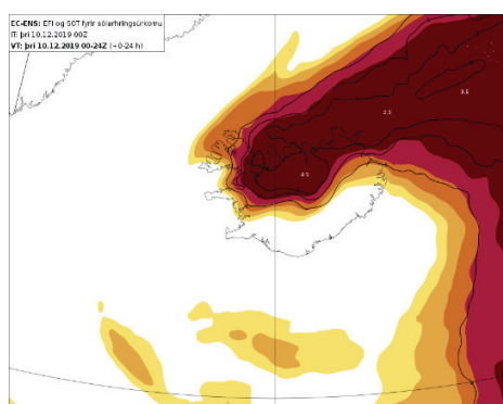
Mynd 16: Aftakaveðurvisir (EFI) og halavísir (SOT) fyrir úrkomu úr EPS spám ECMWF þann 10. desember, EFI og SOT yfir 1 benda til þessa að spáð sé mjög óvenjulegu veðri.
